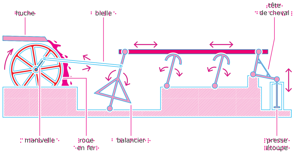
Schéma de la pompe profonde, 19 e siècle
